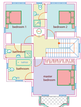
MAISONNETTE FIRST FLOOR PLAN
